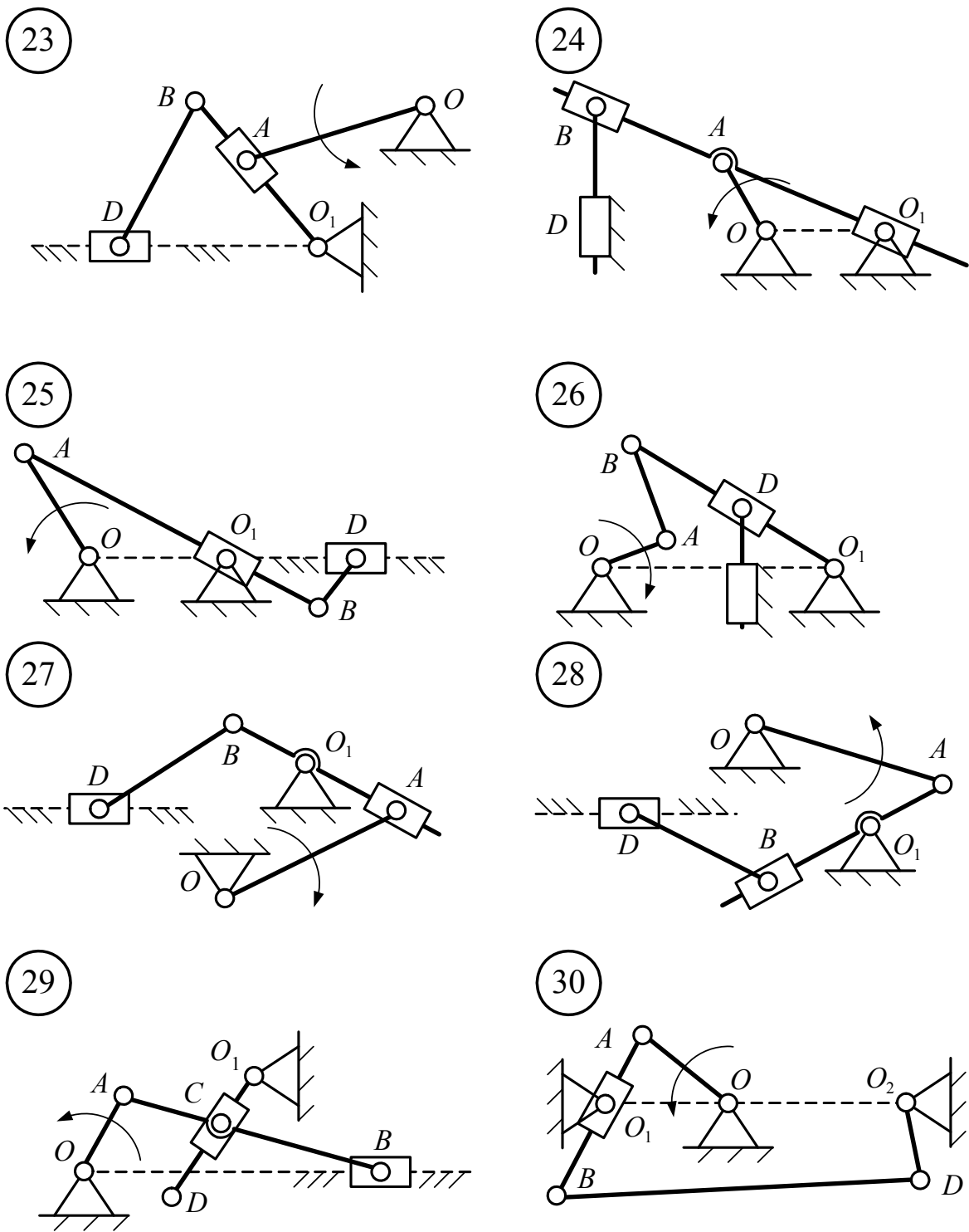
Рис. 1.10. Окончание. Схемы 23–30
