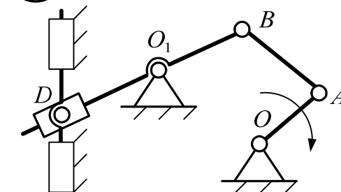
Рис. 1.10. Продолжение. Схемы 7–14
