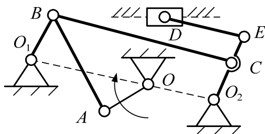
Рис. 1.10. Продолжение. Схемы 7–14
