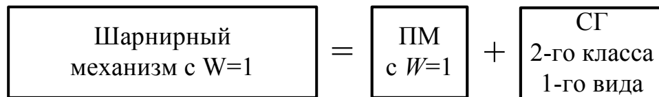
Рис. 1.4. Состав структуры шарнирного механизма
