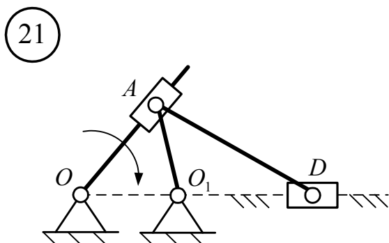
Рис. 1.10. Продолжение. Схемы 15–22
