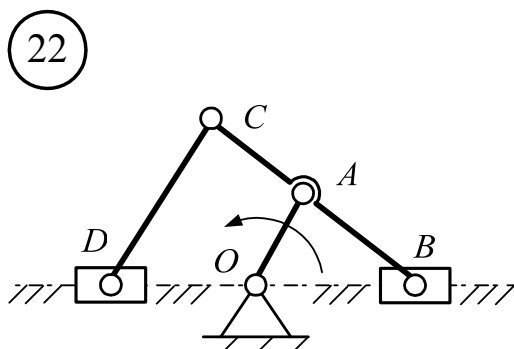
Рис. 1.10. Продолжение. Схемы 15–22
