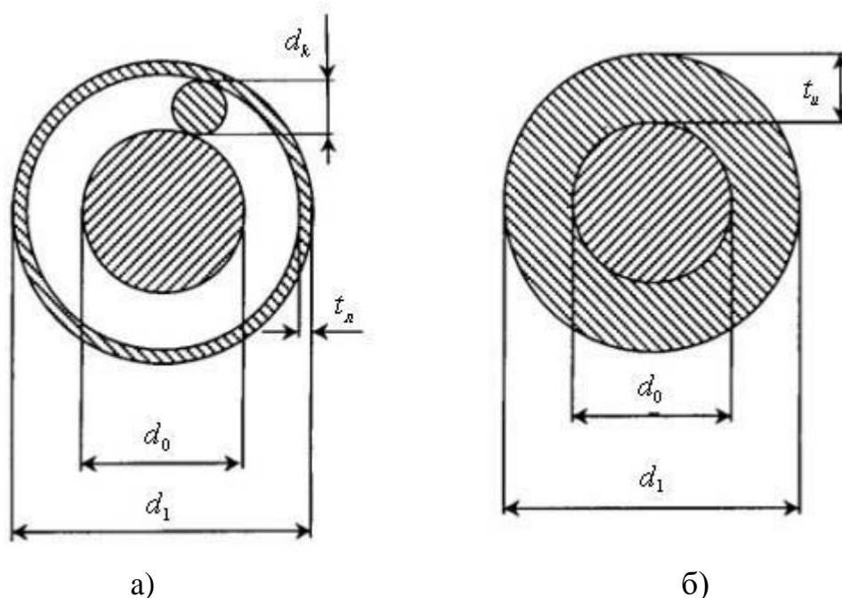
Рисунок 1. Определение диаметра изолированной жилы
